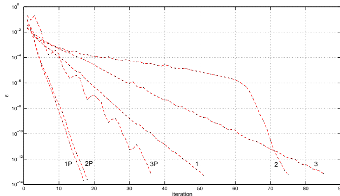
Figure 2. Convergence of the conjugate gradient algorithm for Case 1 , Case 2 and Case 3 with preconditioning (curves 1P, 2P and 3P) and without preconditioning (curves 1, 2, 3). Convergence de l'algorithme de gradient conjugué dans les Cas 1, 2 et 3 avec préconditionnement (courbes 1P, 2P et 3P) et sans préconditionnement (courbes 1, 2 et 3).
