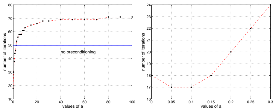
Figure 3. Influence on the number of iterations of the constant a in the Robin condition verified by \varphi . Influence sur le nombre d'itérations de la constante a dans la condition de Robin vérifiée par \varphi .
